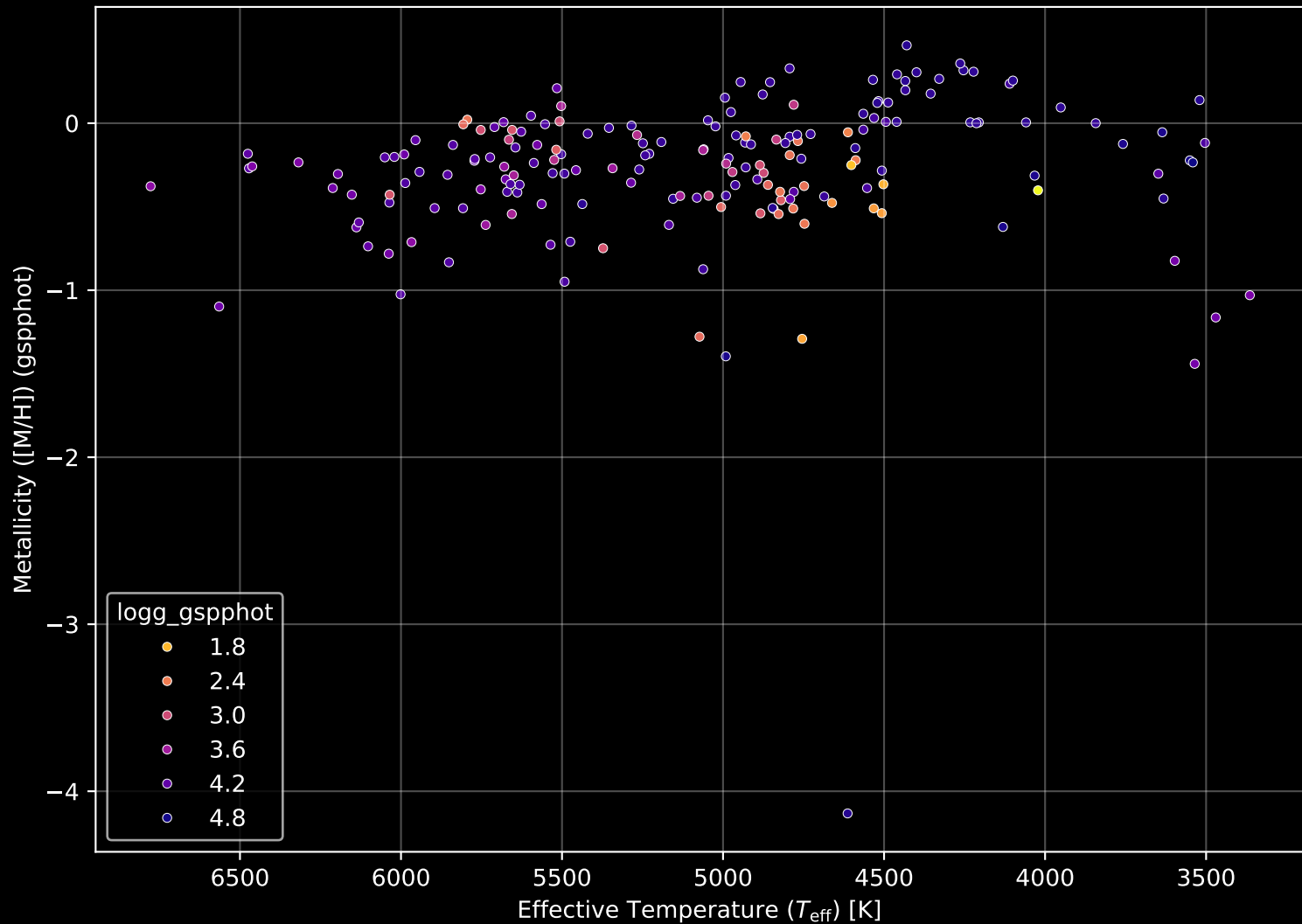
APOGEE DR17 Field: [246+77_btx] Stellar Population Parameters (n= 188)
